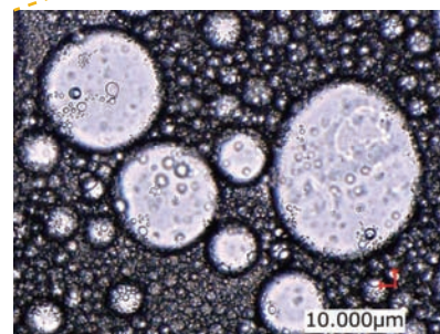
SMD-70乳化装置使用 顕微鏡観察写真×500倍
